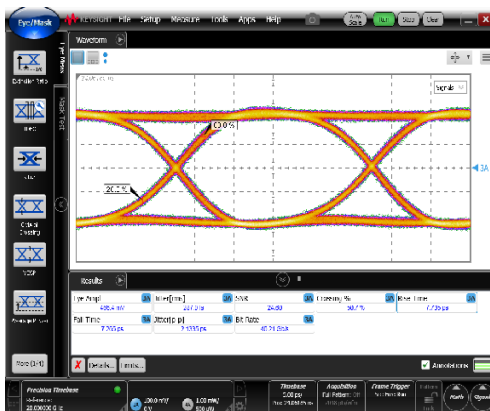
Input signal Eye amplitude = 0.45\text{ V}_{pp}
